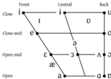
English Vowel
